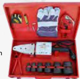
BWM3063 022909 Συγκολλητικό Σωλήνων • Ισχύς 1500W • Διάμετρος σωληνών Ø20-63mm • Με εξαρτήματα
